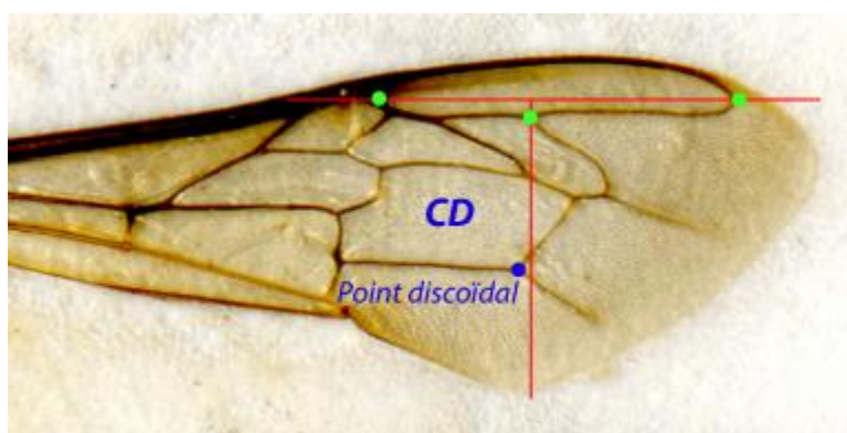
Figure 2 - Aile antérieure de l'abeille et mesure de la transgression discoïdale (ici, la transgression est positive)
